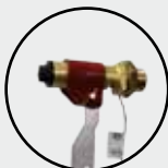
Manchette chauffante (réf. 131.0527) pour la protection antigel élevée de la soupape
