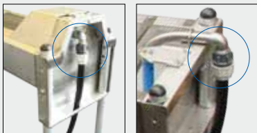
Exemple de montage avec coude inox (accessoires) et tuyau avec raccords PE:
