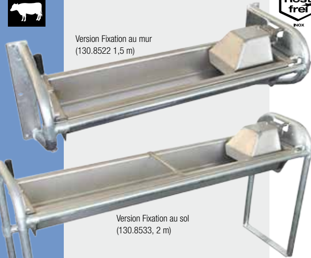
Accès au flotteur par capot relevable, sans outils
