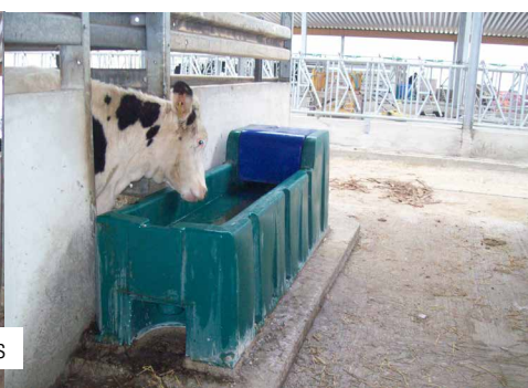
Option H: 1 flotteur MAXIFLOW (sur un circuit en boucle, avec un câble chauffant 24 V, 20 W, 2 m), 1 résistance 24 V, 180 W
