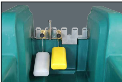
Option D: 1 flotteur MAXIFLOW (jusqu'à 40 l/min !) 1 flotteur basse-pression
