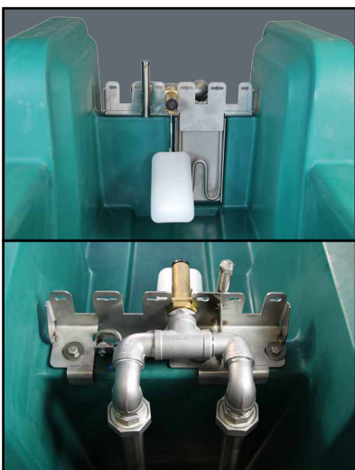
Option G: 1 flotteur MAXIFLOW (monté sur un circuit en boucle) 1 résistance 24 V, 180 W
