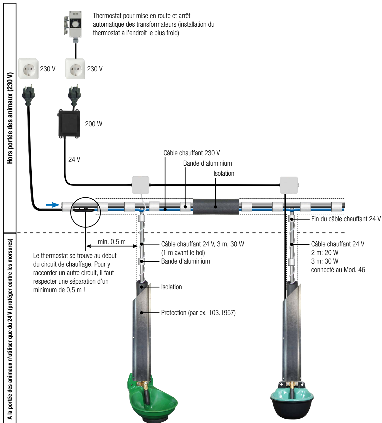
Mod. 12P-HK (voir p. 22) avec bol chauffé en plastique incl. câble chauffant 3 m: 24 V, 30 W = total: 30 W
